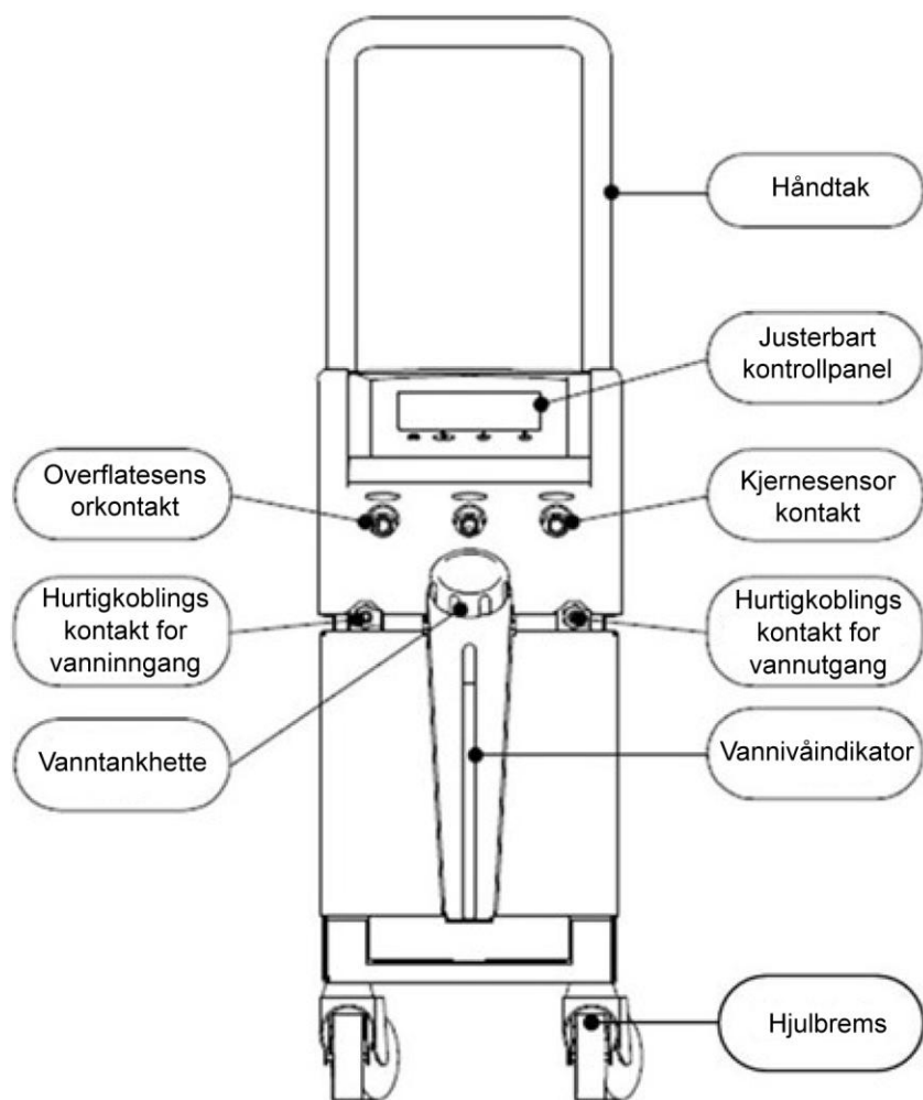
Figur 2: Sett forfra.
