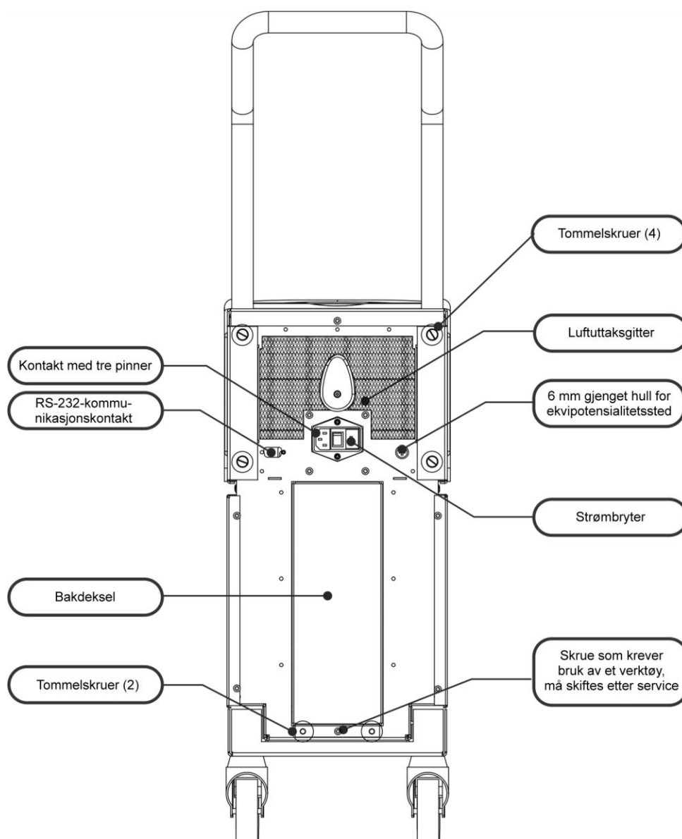
Figur 4: Sett bakfra.
